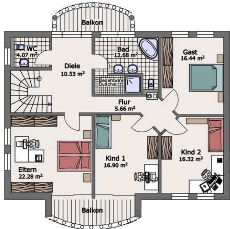
Grundriss DG Wohnfläche 101,7 m 2
